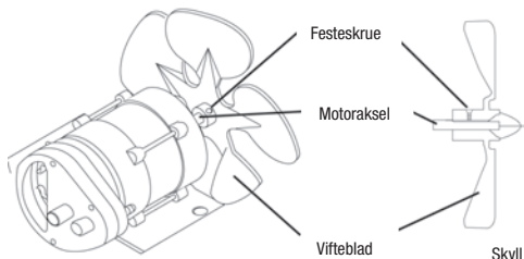
Figur 14: Bytte av vifte
