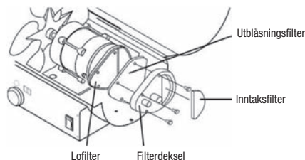
Figur 13: Bytte av filter
